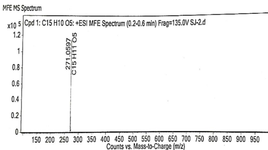
Fig. 2. Mass spectrum of Apigenin (SJ 2)
