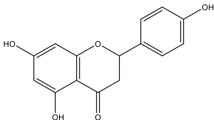
Fig. 1. Apigenin (SJ 2), C_{15}H_{10}O_5 , Mol. Wt: 270.24g/mol
